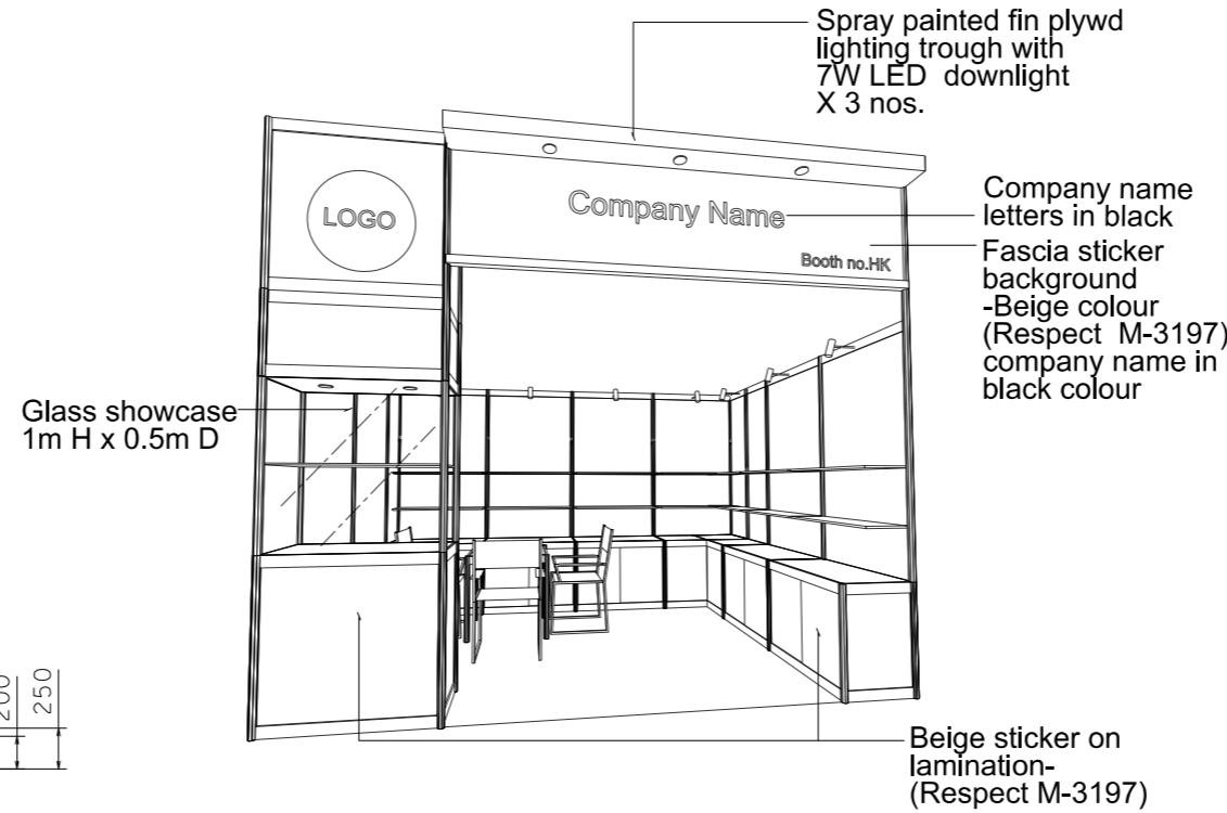
PERSPECTIVE N.T.S
