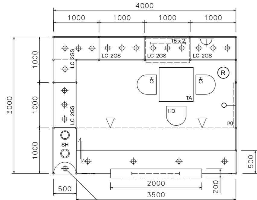
Top Elevation
