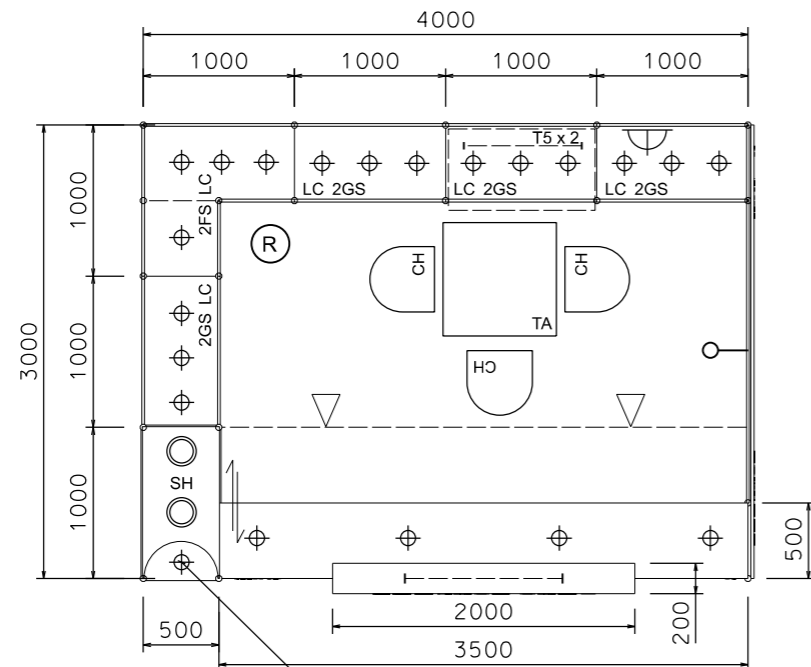
Top Elevation
