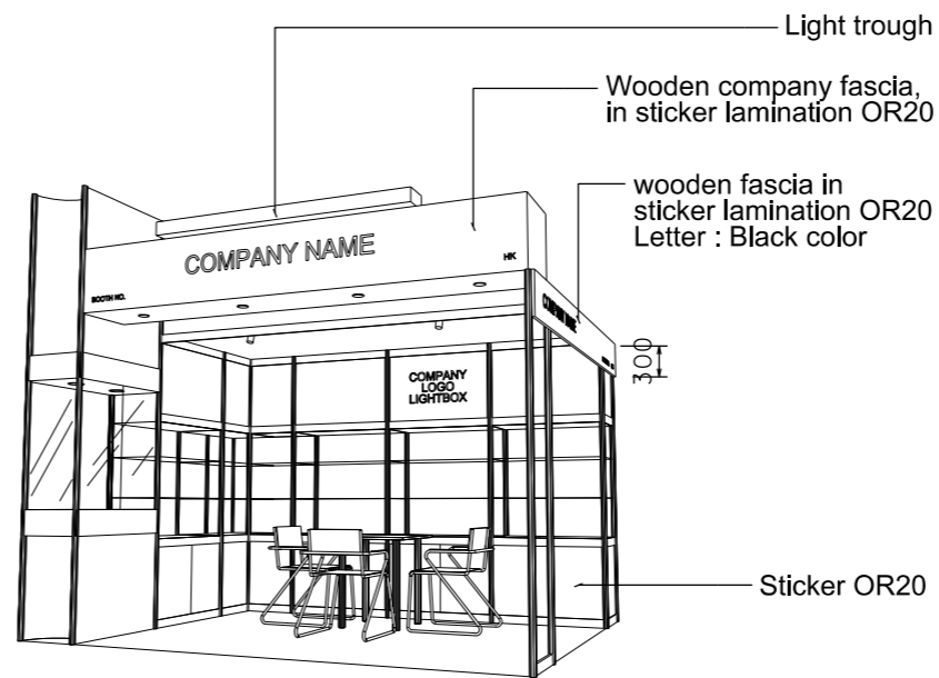
PERSPECTIVE N.T.S
